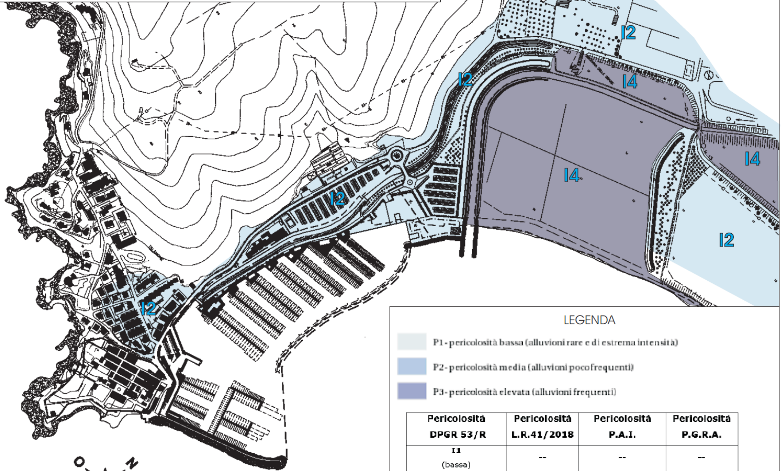
FIG. 20 - Carta della pericolosità idraulica post riconfigurazione foce del canale collettore (Base cartografica: CTR integrato PRP)
