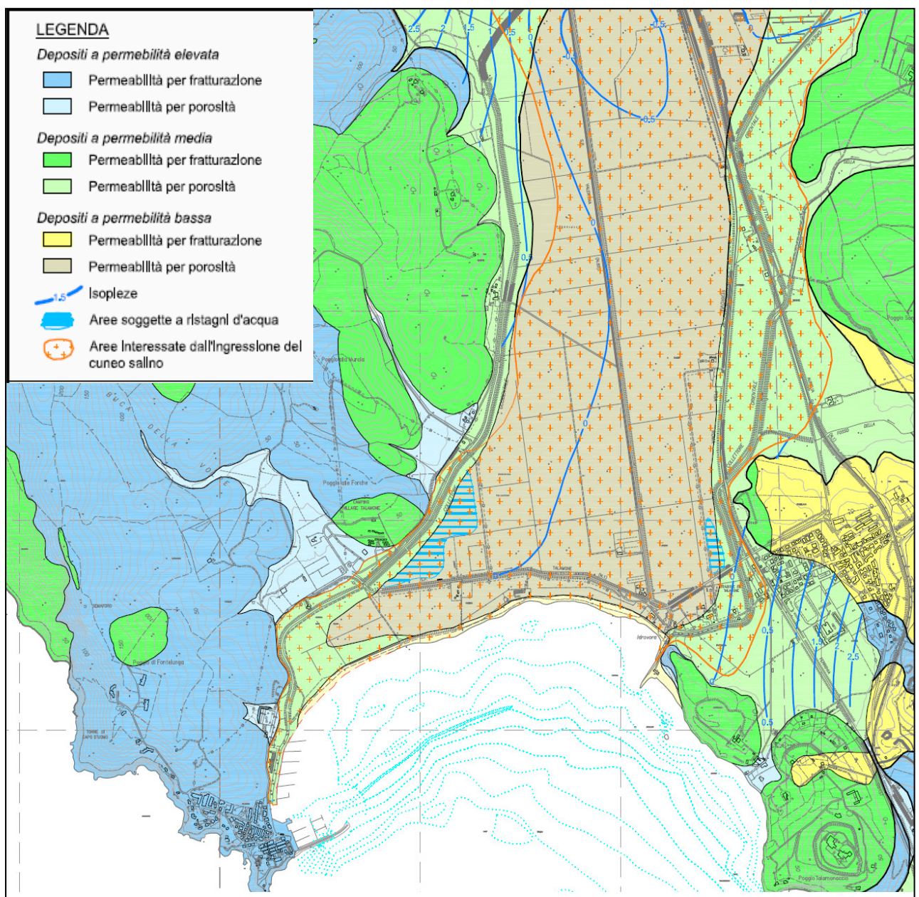
Fig. 4 Carta Idrogeologica (da P.S. Comune di Orbetello modificata)
